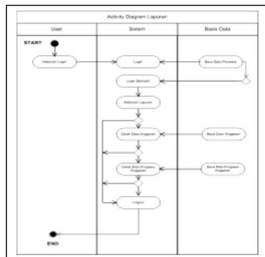
Actifity Diagram Laporan
