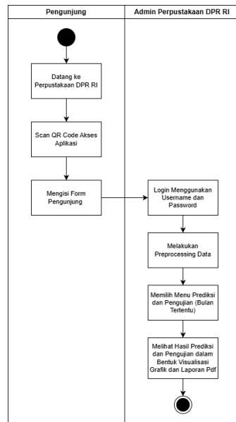
Gambar 1. Analisa Sistem Usulan
