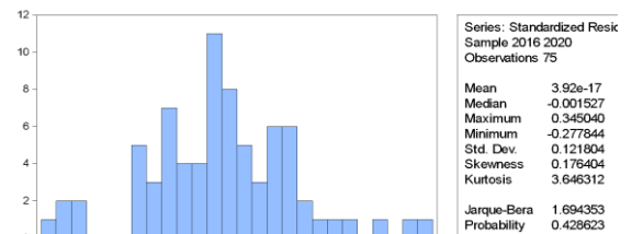
Gambar 1. Uji Normalitas
