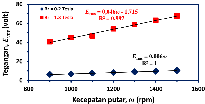
Gambar 11. Hubungan antara output tegangan ( E_{rms} ) generator terhadap kecepatan putar ( \omega ), pada air gap ( L_G ) = 7 mm, dan remanensi, B_r = 0,2 dan 1,3 Tesla.
