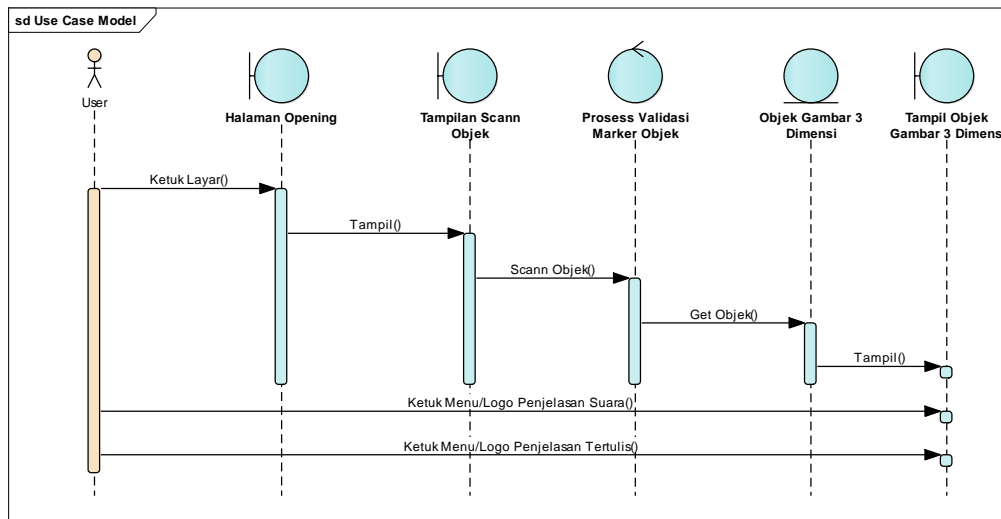
Gambar 5. 5 Squence Mengelola Menu
