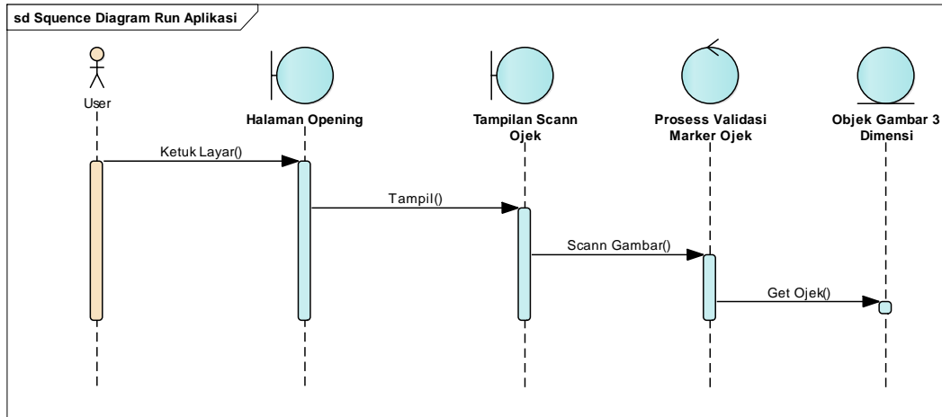
Gambar 3. 4 Squence Menjalankan Aplikasi
