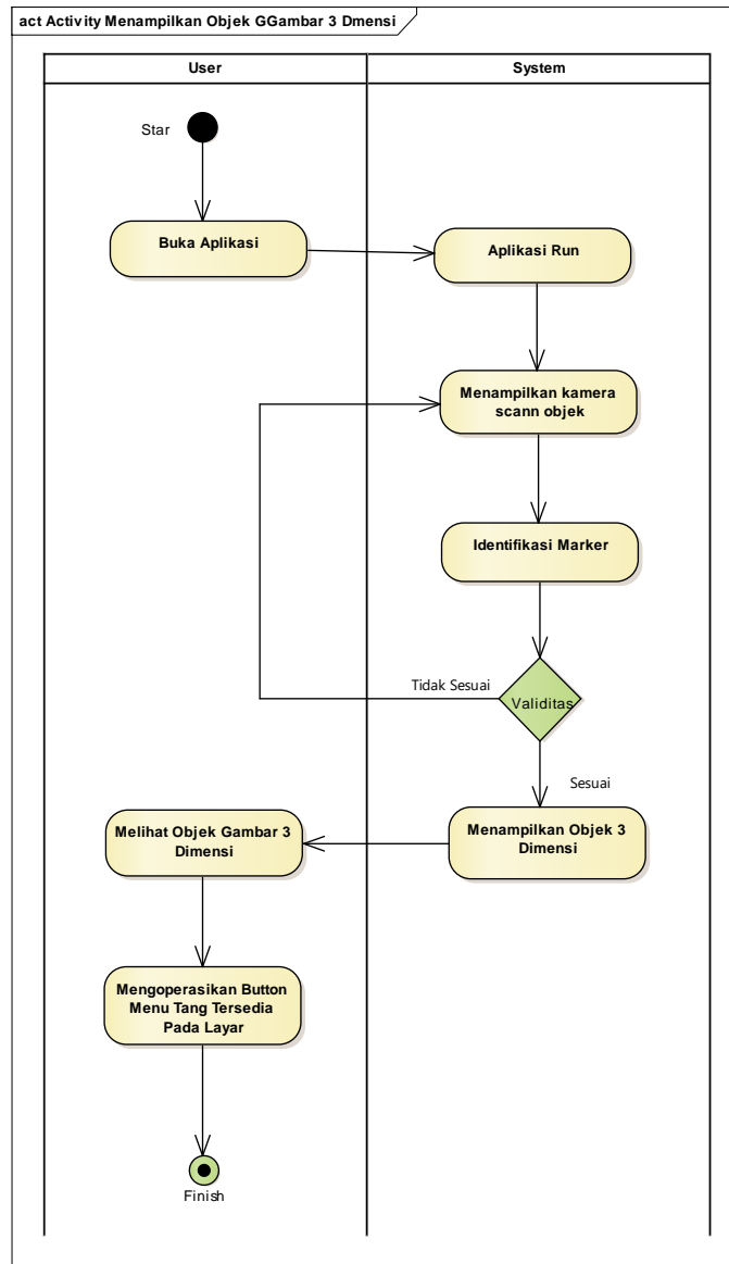
Gambar 3. 3 Activity Membuka Objek Aplikasi
