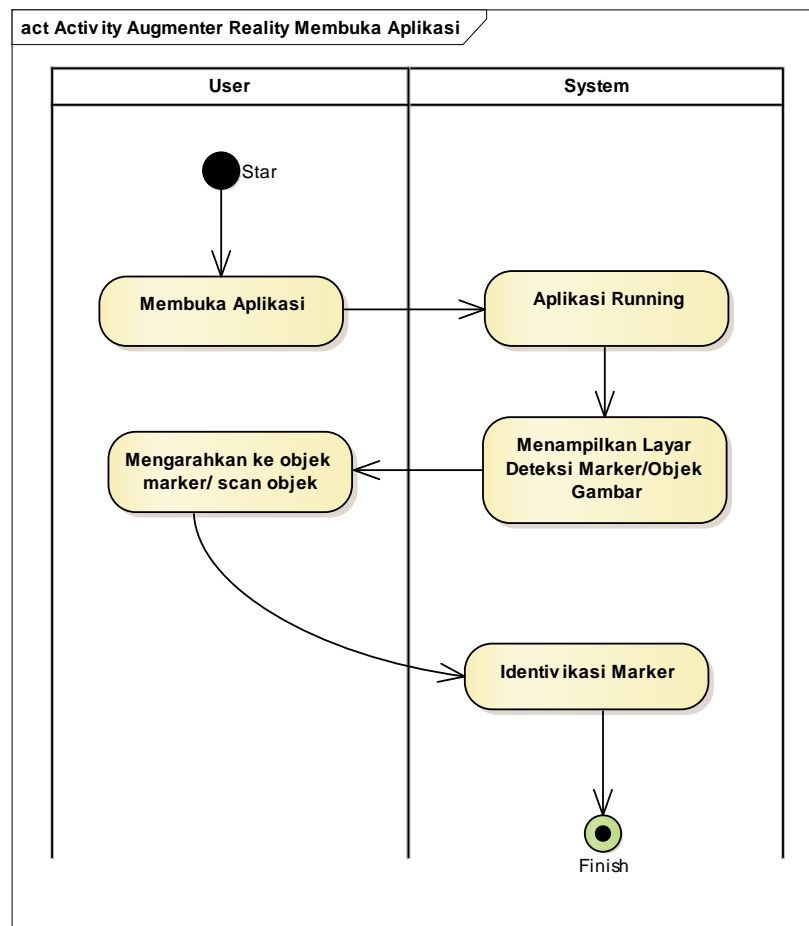
Gambar 3. 2 Activity Membuka Aplikasi
