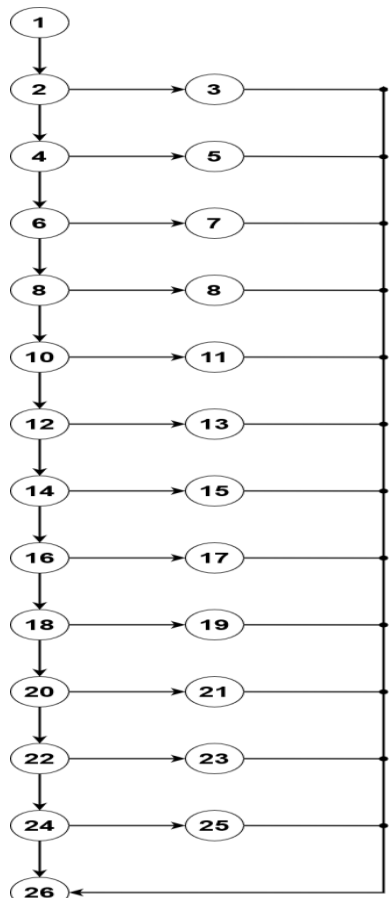
Gambar 1 flow graf fungsi bulan
