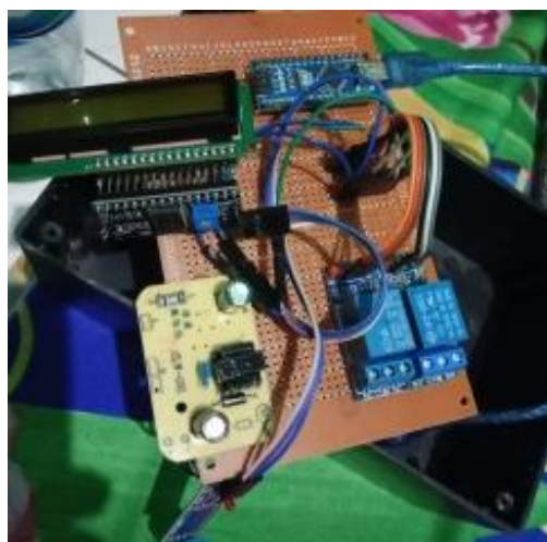
Gambar 7. Rangkaian Alat Prototype
