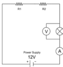
Gambar 2. Rangkaian Seri Resistor
