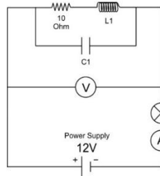
Gambar 6. Rangkaian Seri-Paralel RLC
