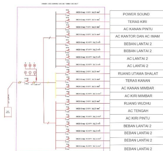
Gambar 5. Single Line Diagram Pembagian Daya Masjid Baitussalam
