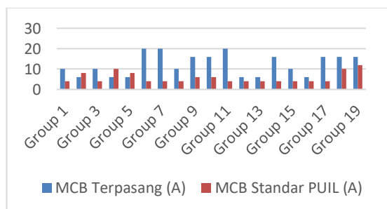
Gambar 25. Perbandingan Nilai Rating MCB yang Terpasang dengan MCB standar PUIL 2011
