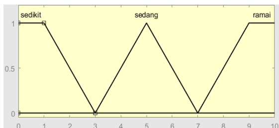
Gambar 8. Fungsi keanggotaan jumlah kendaraan motor
